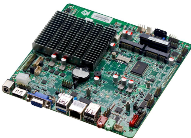
ITX-B190_D912L VER:1.0 主板侧面图
